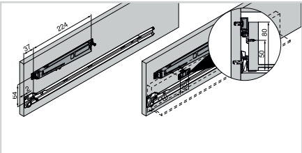
Установочные размеры BLUMOTION для STANDARD
