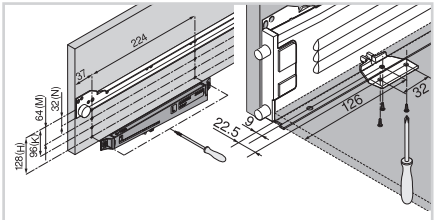
Установочные размеры BLUMOTION для METABOX
