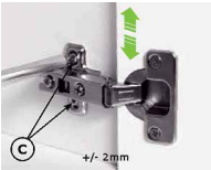
Вертикальная регулировка Поворачивая винт «С» на монтажной планке, возможна регулировка двери по вертикали.
