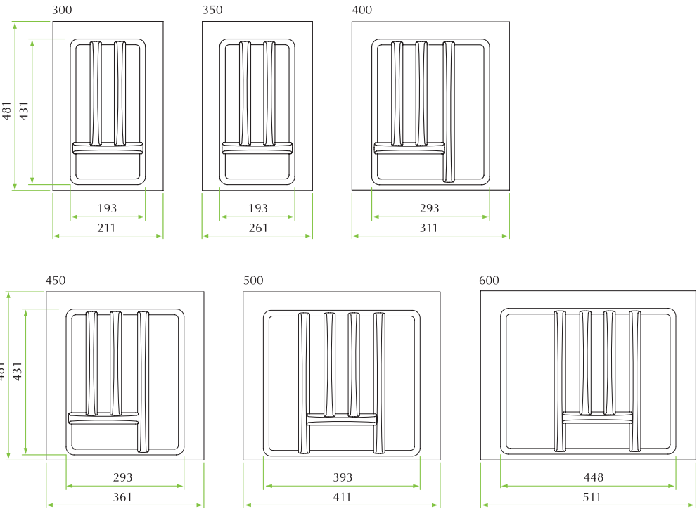
Комбинация органайзера Volumix ящика для оптимизации управления пространством внутри ящика до 600мм
