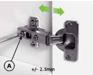
Регулировка фасада Поворачивая винт «А», возможна регулировка расстояния между боковиной шкафа и дверью.
