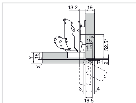
Дверь с фальцем внутренней кромки
