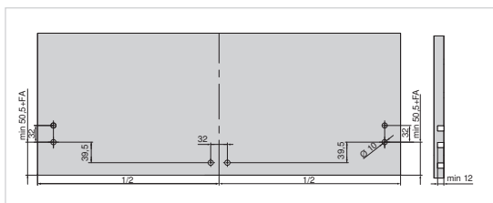
Позиции сверления фасада под уголок, поддерживающий дно
