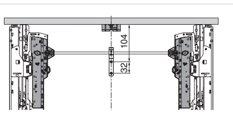
Механизм TIP-ON BLUMOTION, тип L1, L3, L5 (NL ≥ 350–650 мм)
