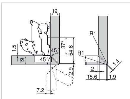
Конструкция встык
