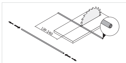
Схема раскроя вала синхронизатора TIP-ON BLUMOTION LW — внутренняя ширина корпуса
