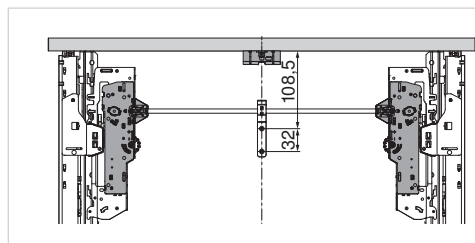
Механизм TIP-ON BLUMOTION, тип S0, S1 (NL < 350 мм)
