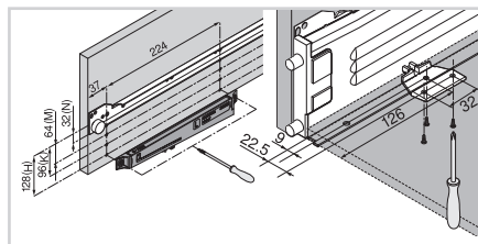
Установочные размеры BLUMOTION для МЕТАВОХ
