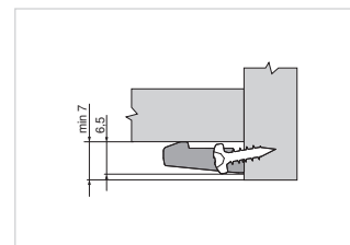
Необходимое пространство в корпусе для уголка, поддерживающего дно
